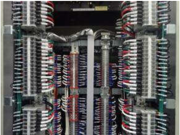
保護リレー装置の裏側（端子台）
