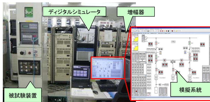
＜デジタル模擬送電線設備＞
