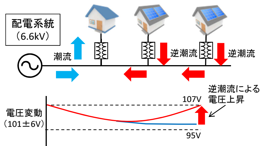
逆潮流に伴う配電系統の電圧上昇(概要)
