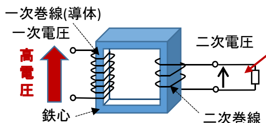
電磁誘導作用を利用した変圧器形(VT)
