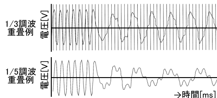
b) 鉄共振発生時のVT二次電圧波形例
