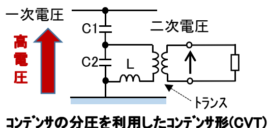
a) VTおよびCVTの原理
