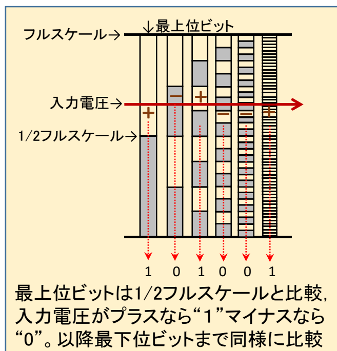
a) デジタル化の概念図
