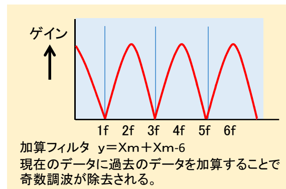
a) デジタルフィルタのアルゴリズム例
