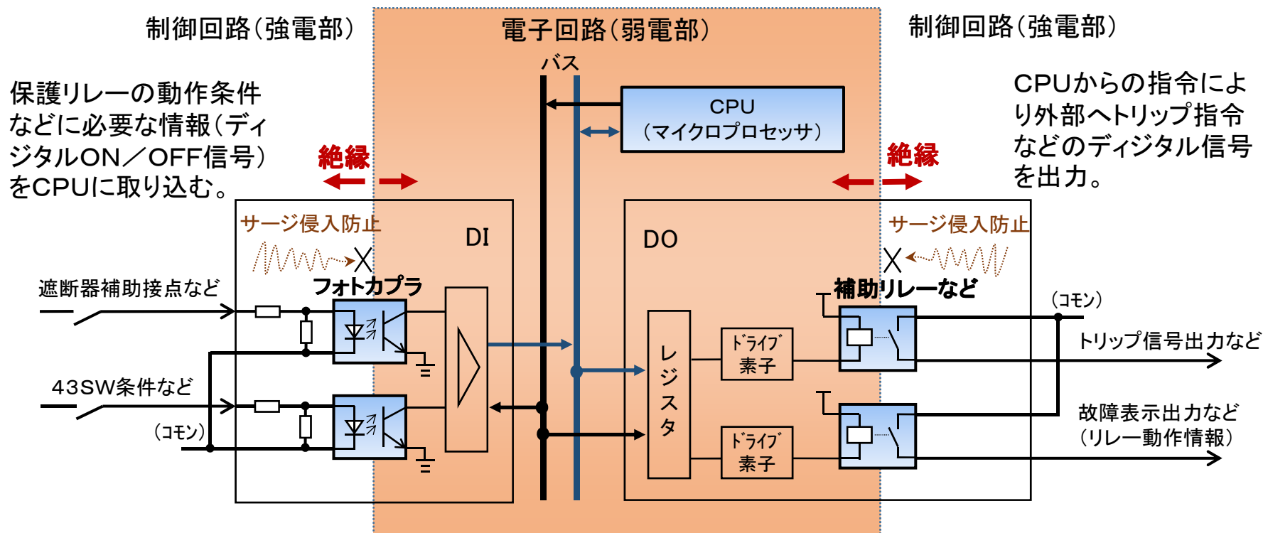
a) DI/DO部の概略構成例
