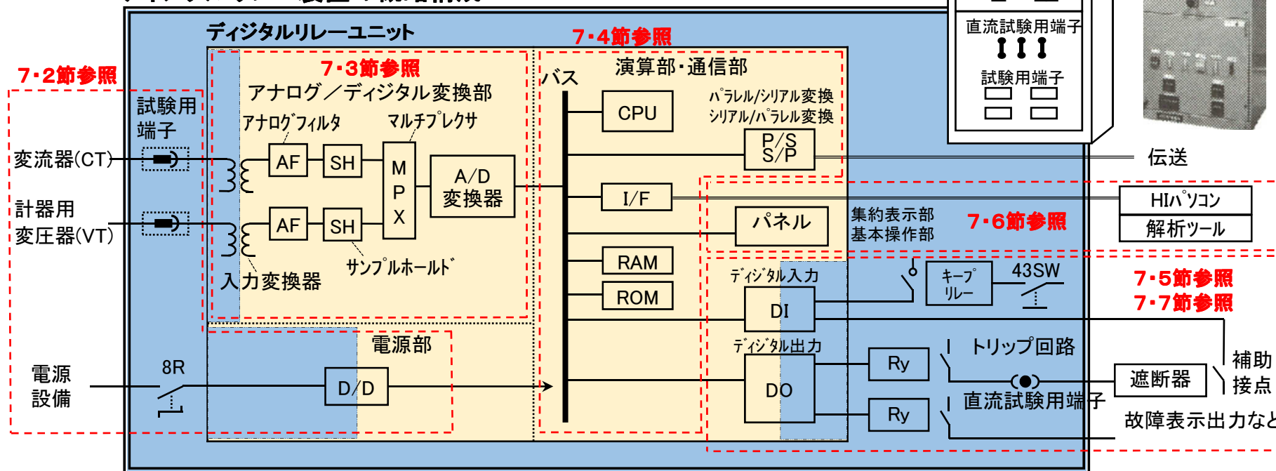
デジタルリレー装置の概略構成
