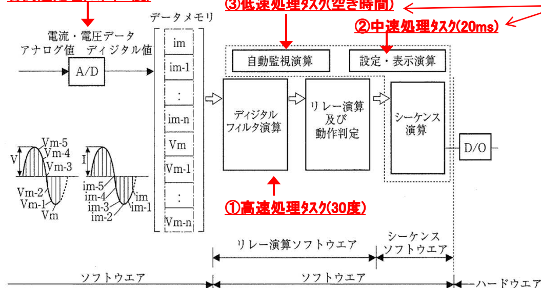
a) ソフトウェア構成例
