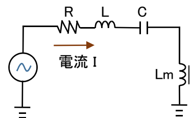
a) 鉄共振現象の基本回路
