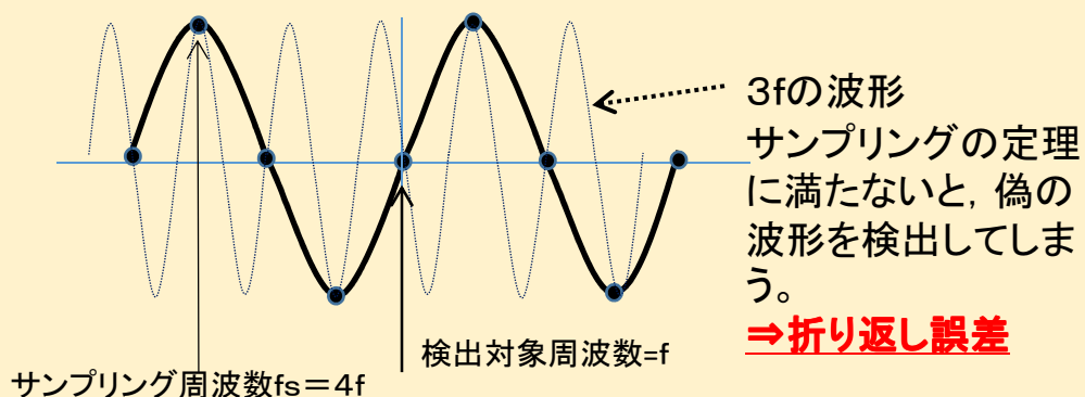
b) 折り返し誤差の例
