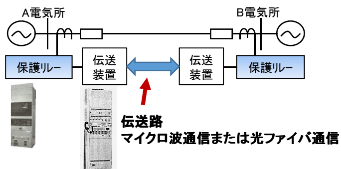
a) キャリアリレー方式の構成と伝送路
