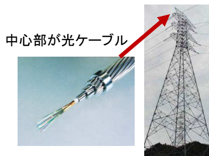
b) OPGW方式の光通信
