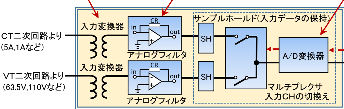
アナログ／デジタル変換部の概略仕様
