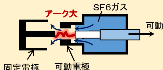
a) ガス遮断器(GCB)の内部構造イメージ図
