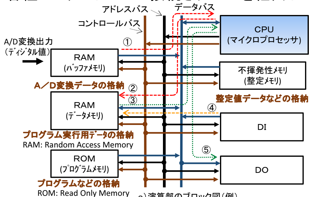
a) 演算部のブロック図 (例)
