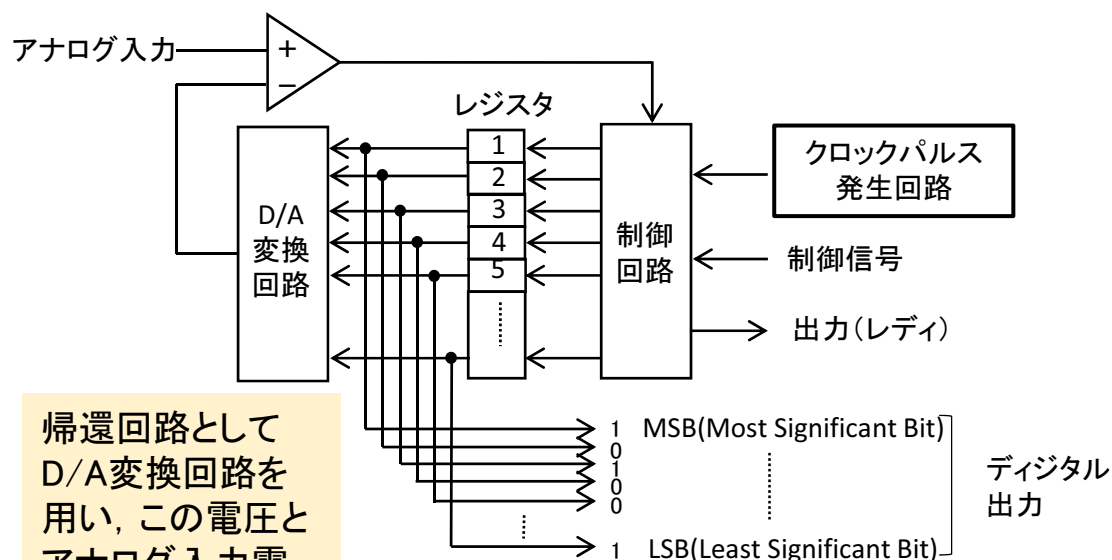
b) A/D変換の方法(代表例: 逐次比較形)
