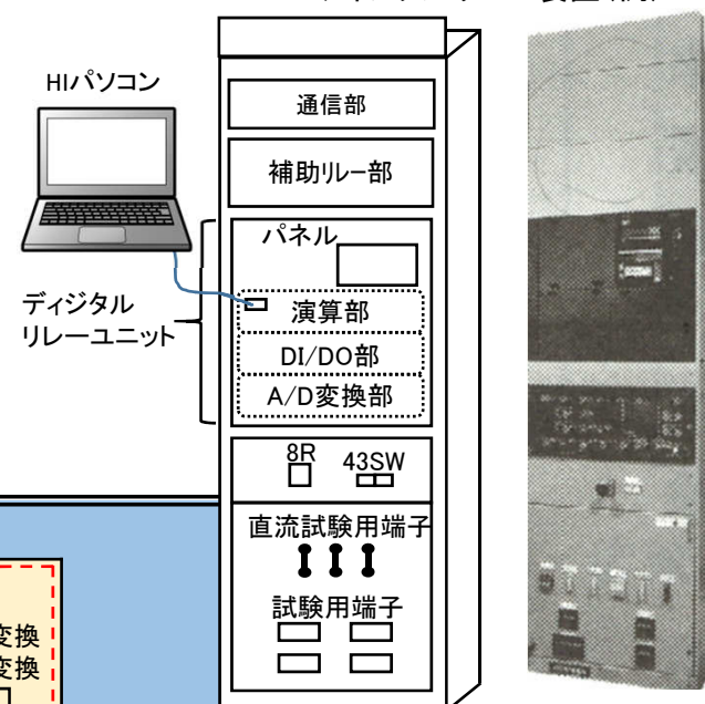
デジタルリレー装置（例）
