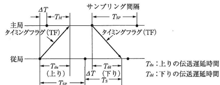
b) サンプリング同期制御の方法
