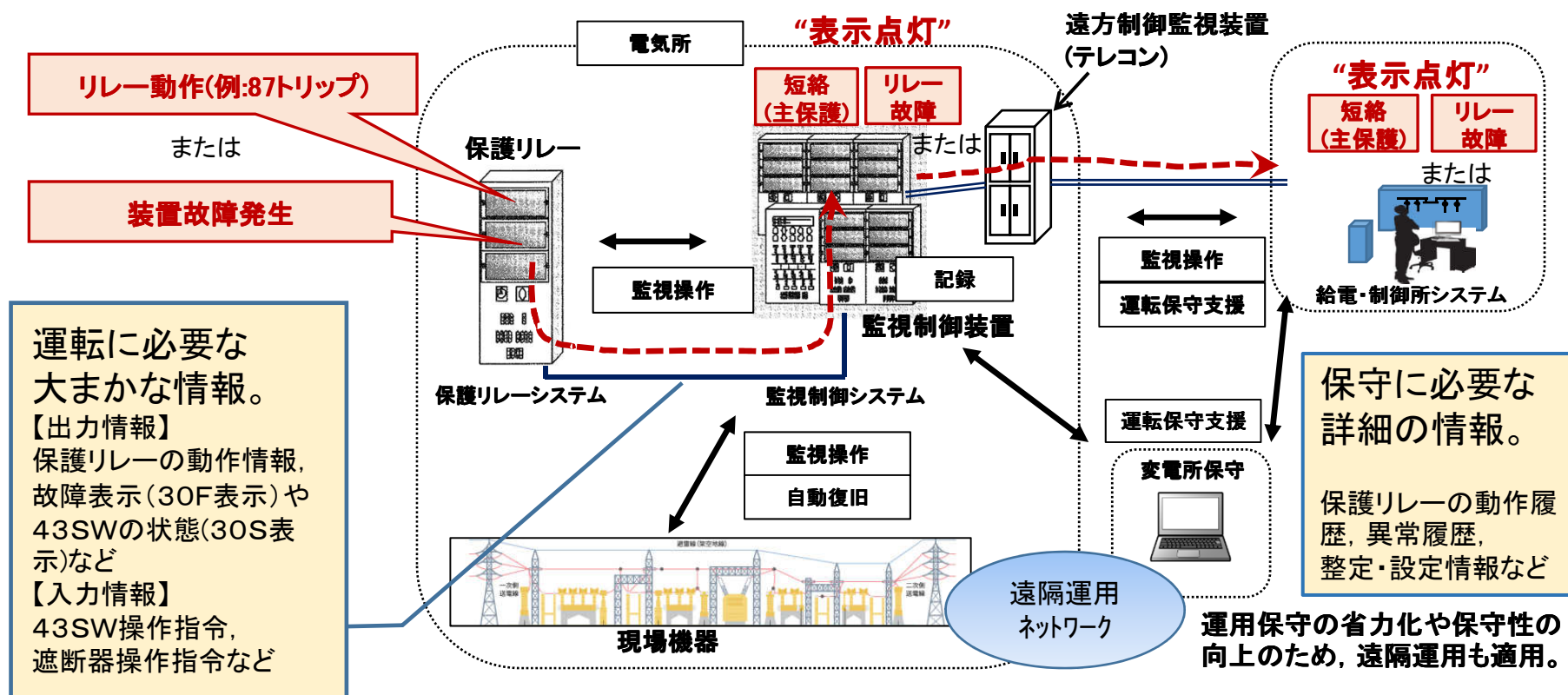
a) 保護リレーシステムと変電所監視制御システムの構成例
