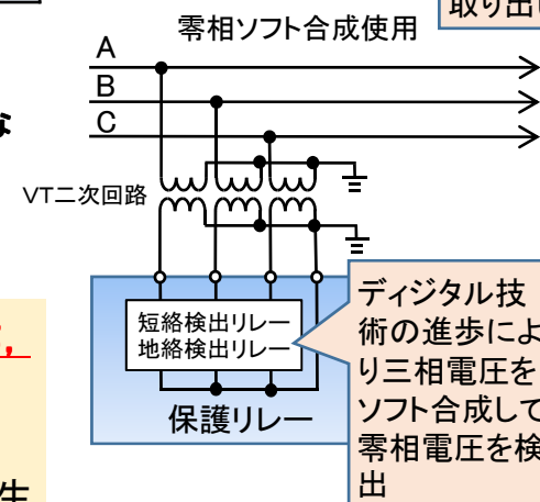
b) VTの結線方法代表例
