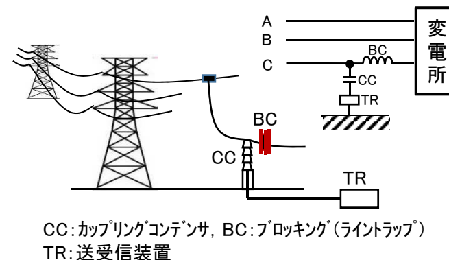
c) 電力線搬送方式における伝送方式例
